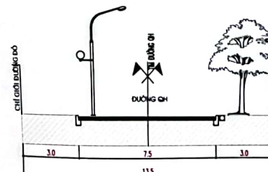
MẶT CẮT 2 - 2
