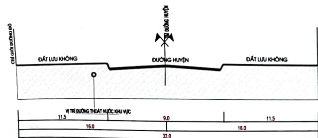
MẶT CẮT 1 - 1
